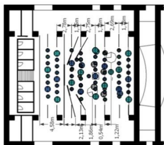
01_Planta
